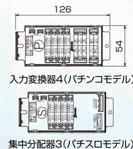
入力器寸法図 (mm)
