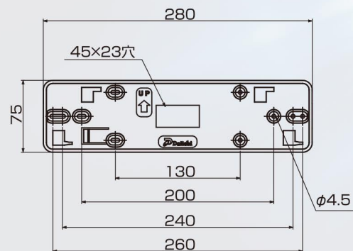
取付ベース寸法図 (mm)
