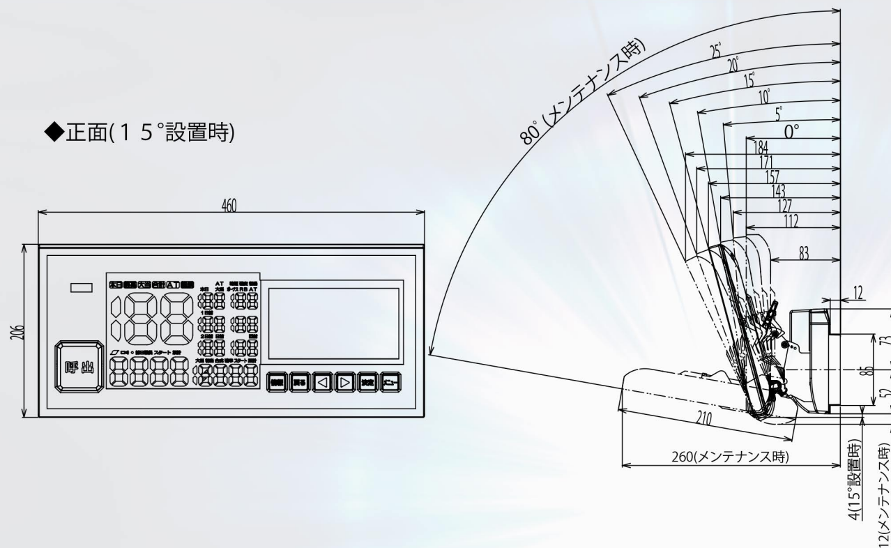
本体外形寸法図 (mm)
