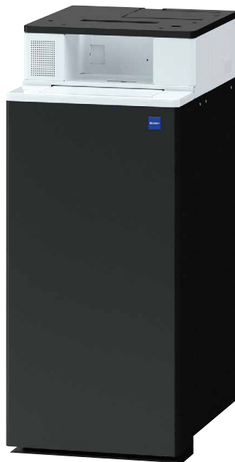
《マルハン清河寺店》のセルフカウンター。賞品払出機はコンパクトサイズの『JK-C500』を使用。設置場所を選ばず、営業スタイルに合わせて自由に設置できる点が特徴。賞品の取り忘れがなく、在庫の補充なども簡単だ。
